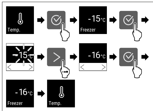
Fig. 68 Cambio de temperatura de -15 °C a -16 °C
