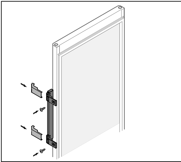
Fig. 25 Porte vitrée*
